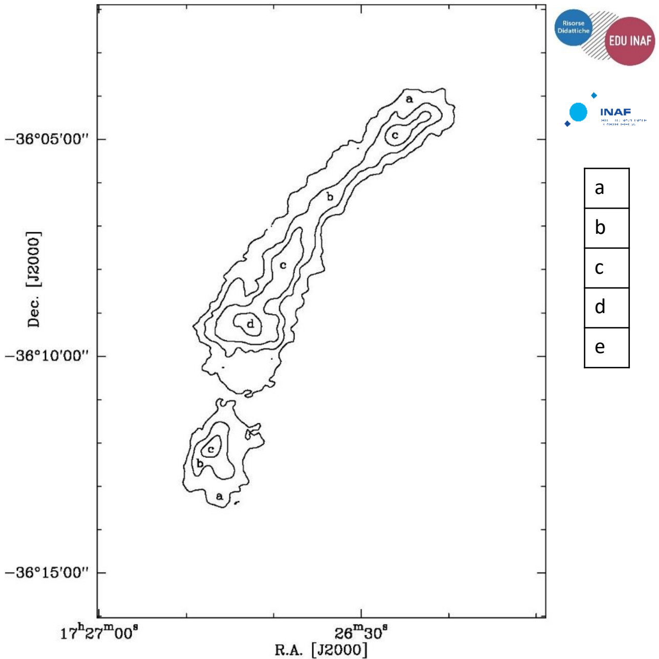
Mappa della nube molecolare G351.776-0.527 , osservata con l'interferometro ATCA (Australia Telescope Compact Array) . Credits: Silvia Leurini (INAF-OACa)
