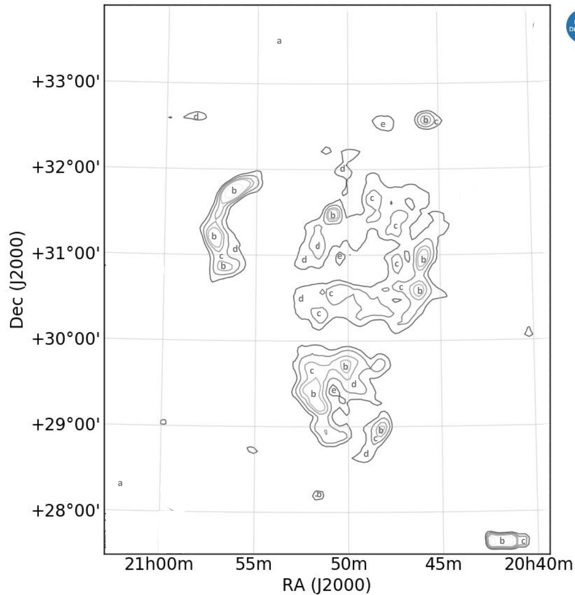
Mappa di Cygnus Loop, osservata con il Sardinia Radio Telescope (SRT) Credits: Sara Loru (INAF-OACT)
