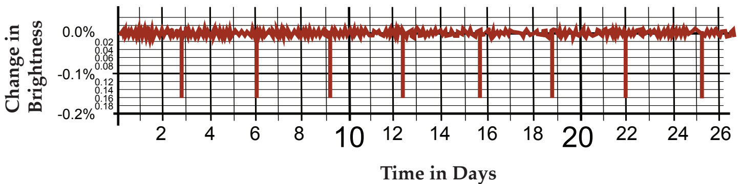
Kepler-4b
