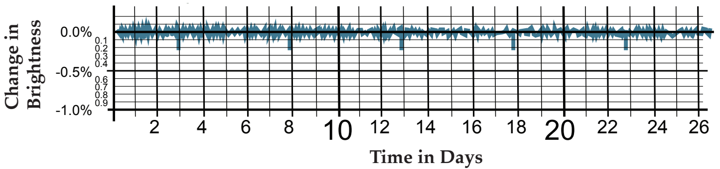
Kepler-4b
